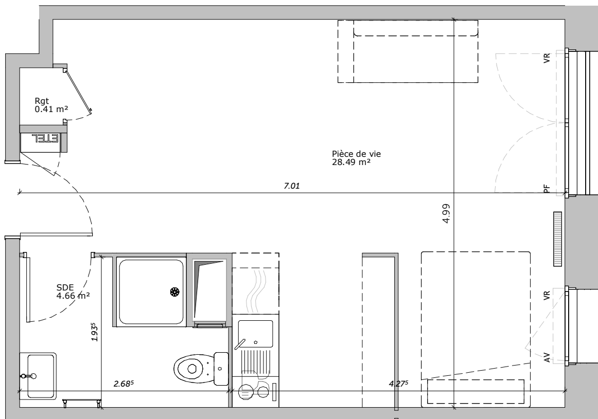
Plan de repérage appartement B-211
