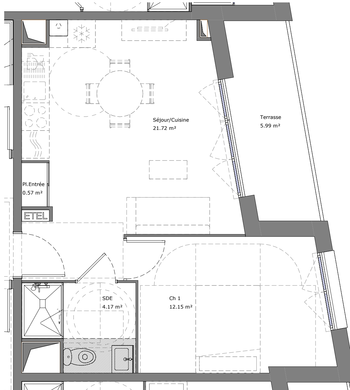
Plan de repérage appartement B_301
