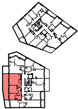
Plan de repérage appartement A_204
